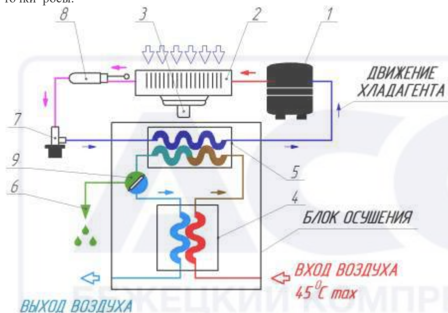
Рисунок 3 Охлаждающий контур
