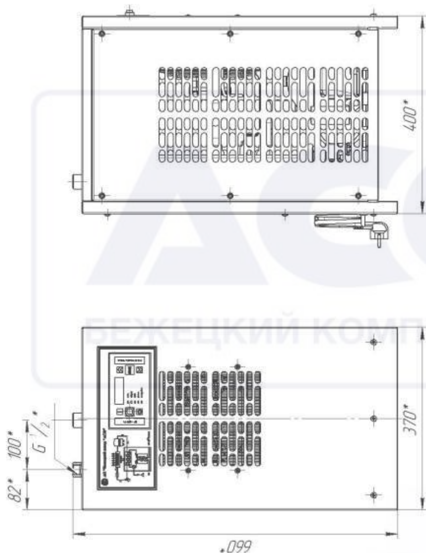
Рисунок 1 Общий вид осушителя
