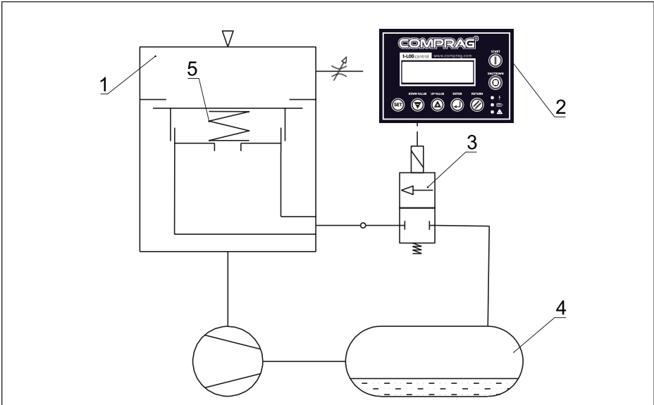
Bild 2.5 Pneumatikplan
