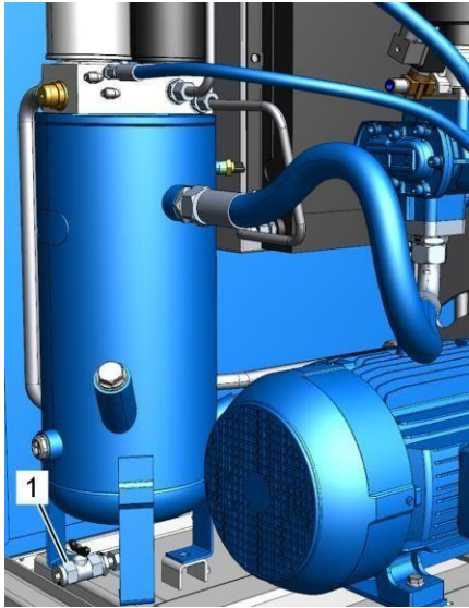
Рис. 44: Отверстие для слива охлаждающей жидкости
