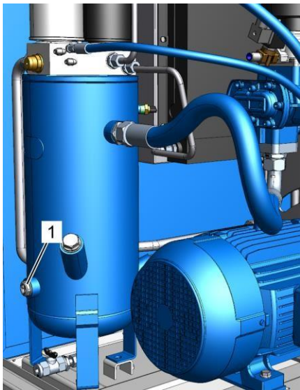
Рис. 39: Смотровое отверстие
